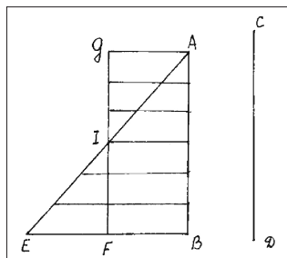
Рис. 27. Пояснительный чертеж Галилея к его рассуждениям о равноускоренном движении (из рукописного троктата De Motu locali ).
