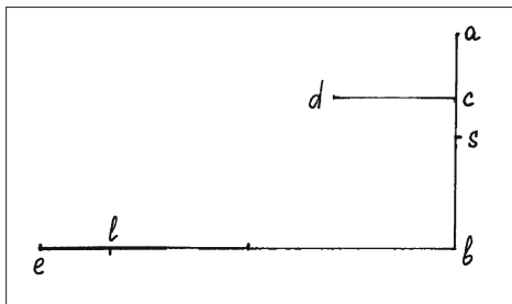
Рис. 22. Диаграмма Галилея к доказательству закона равноускоренного движения ( V \sim t ).
