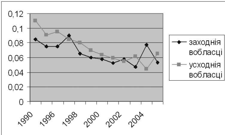
Мал. 21. Дынаміка паказчыка траўматызму на вытворчасці са смяротным зыходам (на 1000 працуючых) па двух заходніх і двух усходніх абласцях Беларусі (прадстаўленыя сярэднія значэнні па рэгіёнах) (1990-2005 г.)
