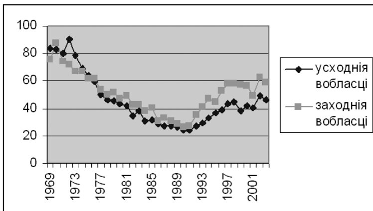
Мал. 25. Дынаміка захворваемасці на сухоты сельскага насельніцтва (на 100 000 нас.) дзвюх заходніх і дзвюх усходніх абласцей Беларусі (1969-2005 г.) (прадстаўленыя сярэднія значэнні паказчыка ў групе)
