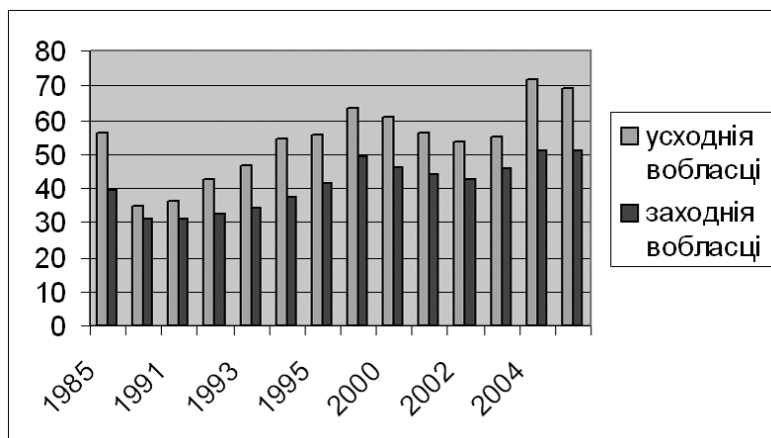
Мал. 23. Сярэдняе значэнне паказчыка захворваемасці на сухоты (на 100000 нас.) у дзвюх заходніх і ў дзвюх усходніх абласцях Беларусі (1985-2005 г.)
