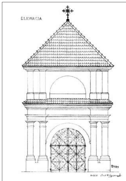
Brama przy kościele Bernardynek. Projekt przebudowy, rys. Bronisław Żywno, 1935 r.
