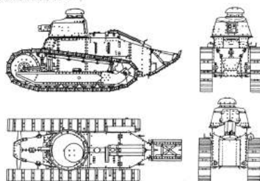
Лесной танк «Рено» FT-17
