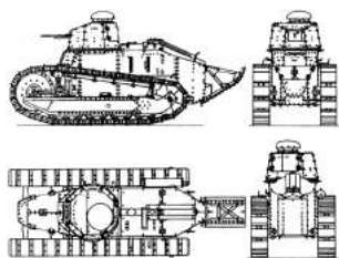
Лесной танк «Рено» FT-17 в пулеметном варианте (Char Mitrailleur 8 mm) с классической башней.
