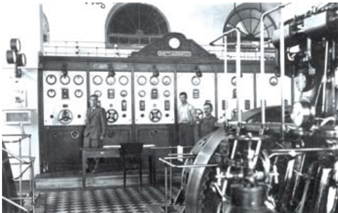
Лідская электроўня пасля рэканструкцыі, машынны зал, на галоўным шчыту надпіс "Ganz"
