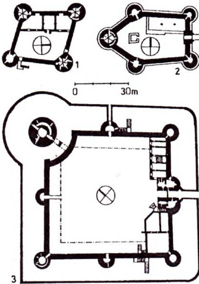
План замка Філіпа II Аўгуста ў Іль-дэ-Франс. 1 — Эўрэ-ле-Шато. 2 — Монлеры. 3 — Дурдан.
