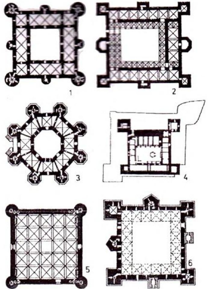
Планы замкаў Фрыдрыху II Штаўфену ў Паўднёвай Італіі. 1 — Кастэль Урсіна ў Каталіі. 2 — Аўгуста. 3 — Кастэль дэль Монтэ. 4 — Трані. 5 — Кастэль Маньяс у Сіракузах. 6 — Прато.
