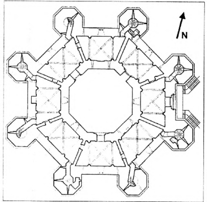
План замка Кастэль дэль Монтэ.
