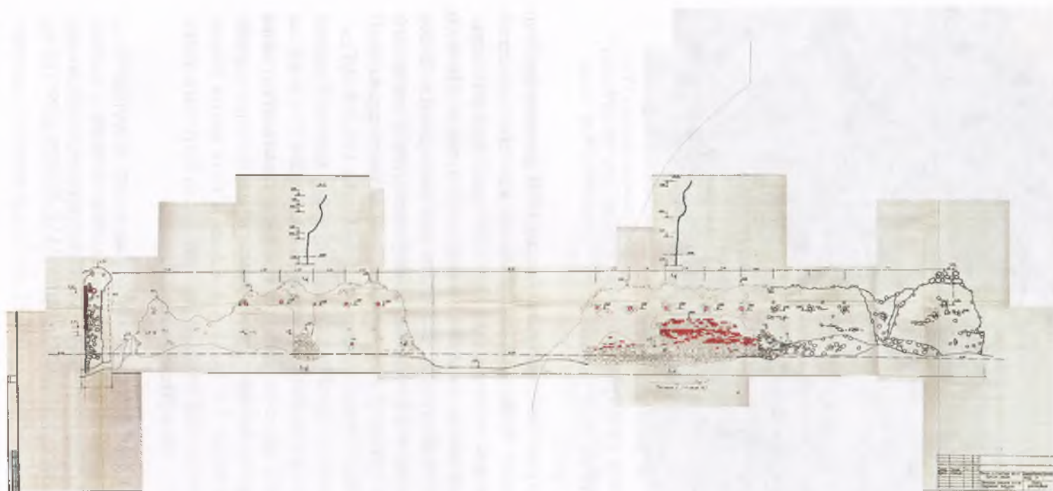
Іл. 24. Абмерны чарцёж паўднёва-заходняй сцяны Крэўскага замка са знешняга боку. Фотаграмметрыя (выканалі Валерый Пінчук і Ігар Русецкі). М 1 : 50. 1994 г.
