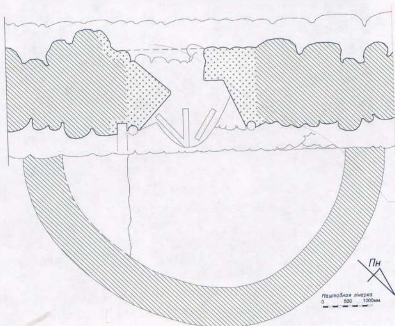
Іл. 17. План ДАКа і амбразуры ў праёме Малой брамы (архітэктар Андрэй Шулаеў)
