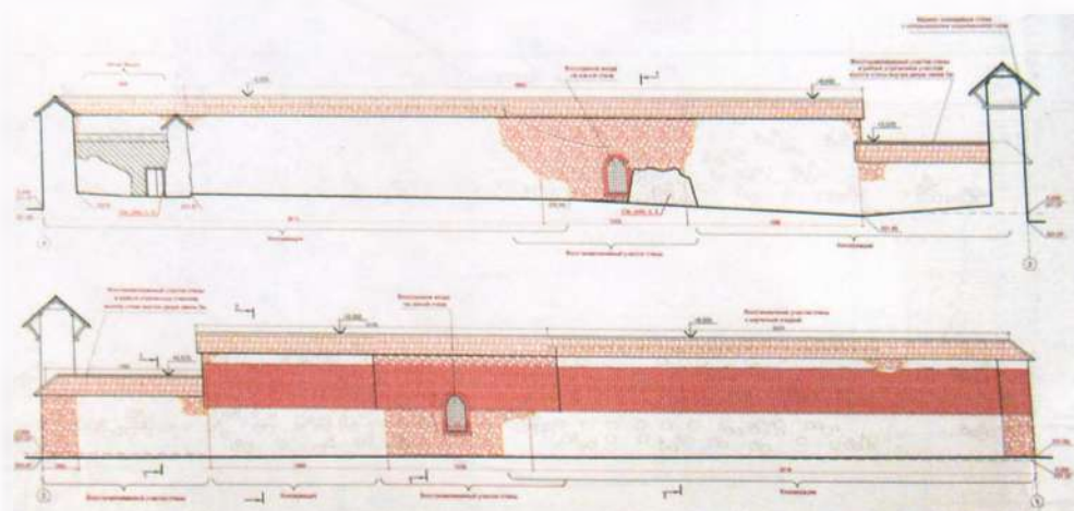
Іл. 30. Першапачатковы практычны варыянт размяшчэння Малой брамы
