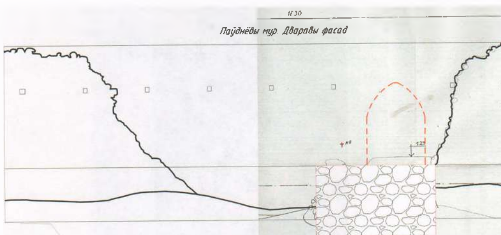
Іл. 29. Фіксацыя захаванага ўзроўню паўднёва-заходняй сцяны Крэўскага замка (чорная лінія) і рэканструкцыя плоскасці сцяны разам з аркай Малой брамы (чырвоная лінія). Пазначаны аб'ём ДАКа. Фасад з боку дзядзінца
