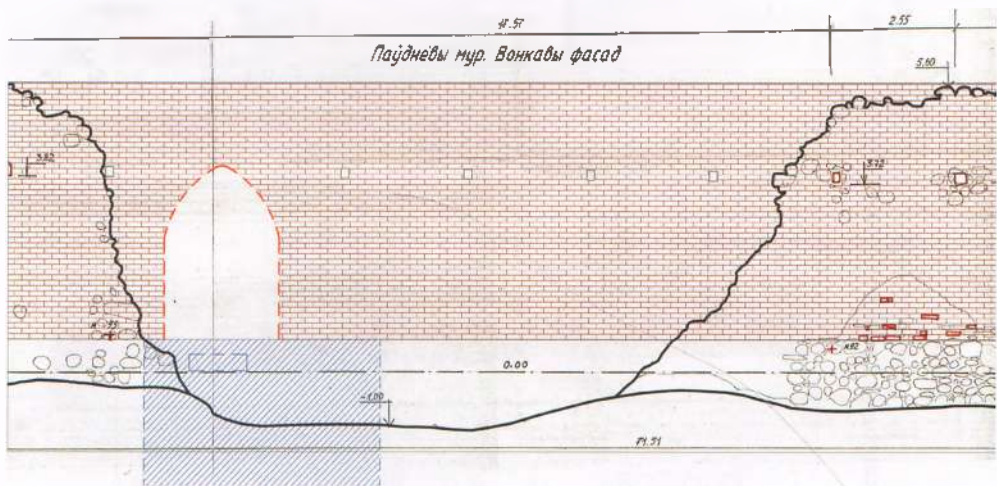
Іл. 28. Фіксацыя захаванага ўзроўню паўднёва-заходняй сцяны Крэўскага замка (чорная лінія) і рэканструкцыя плоскасці сцяны разам з аркай Малой брамы (чырвоная лінія). Знешні бок. Сіняя штрыхоўка – пазначэнне аб'ёму ДАКа
