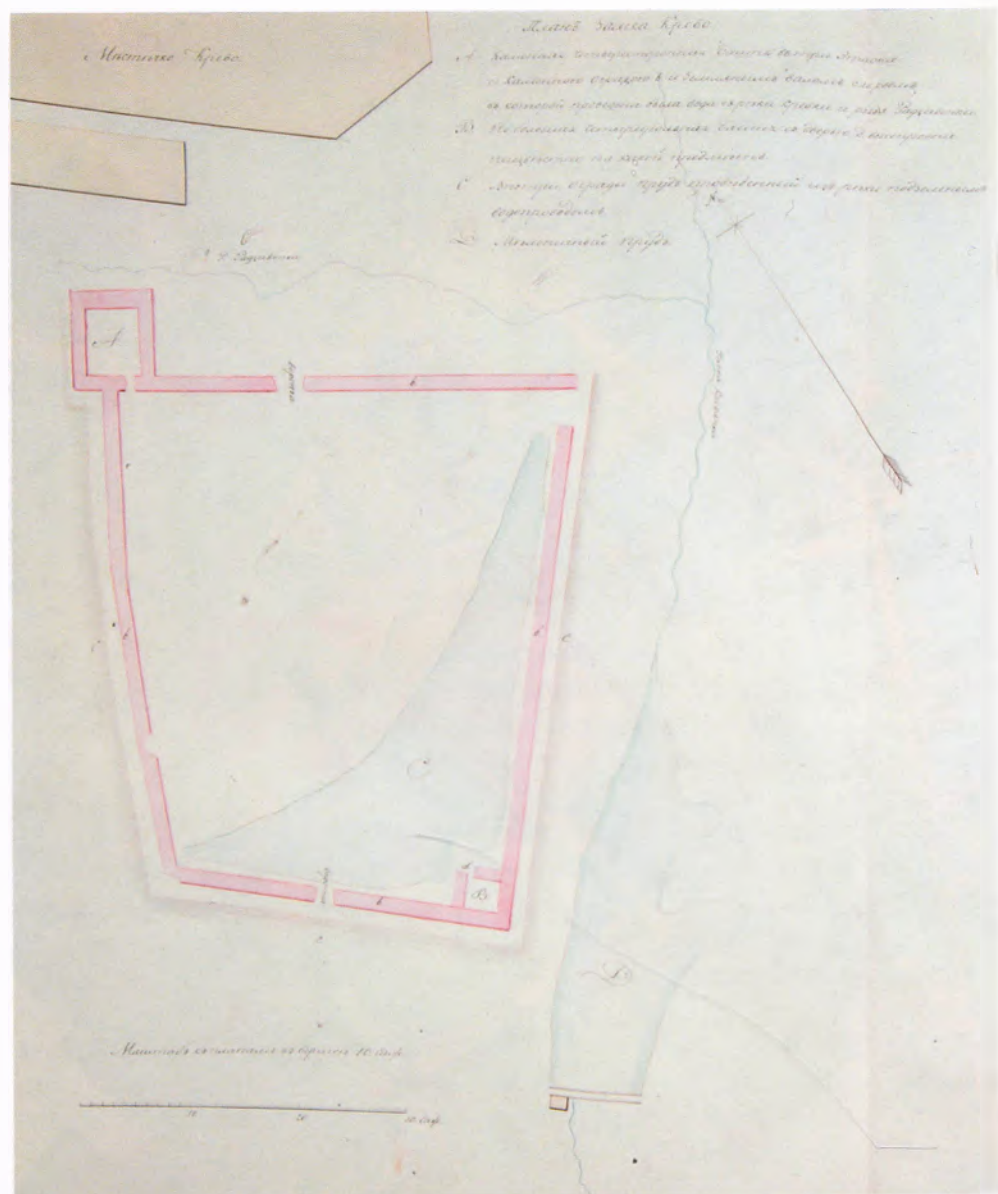
Іл. 2. Крэўскі замак. План 1827 г. («Атлас замков Виленской губернии». Muzeum Narodowe w Krakowie. MNK III-r.a-18320/7)
