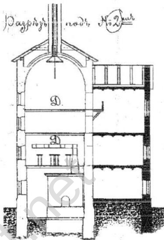
Сушня з комінам Разрз
