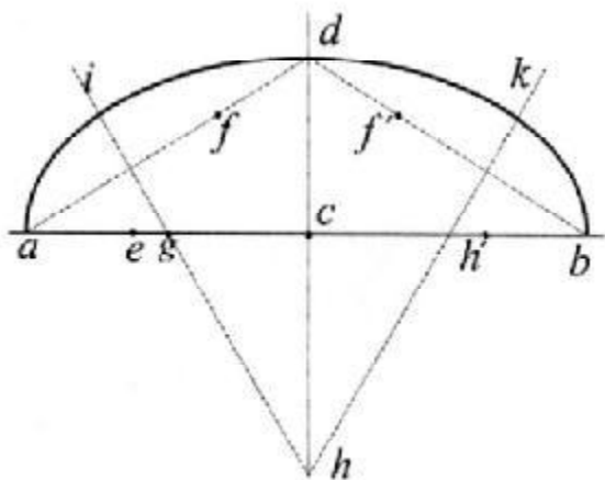
Пабудова скляпення печи
