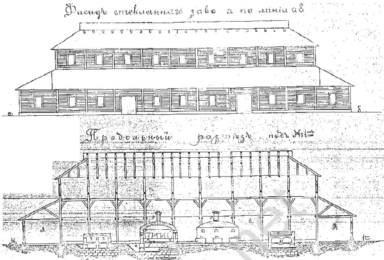
Фасад будинка заводу
