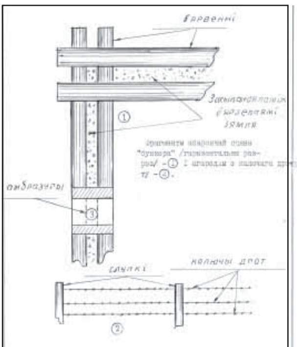
Драўляна-зямельнае абарончае збудаванне - нямецкі бункер.
