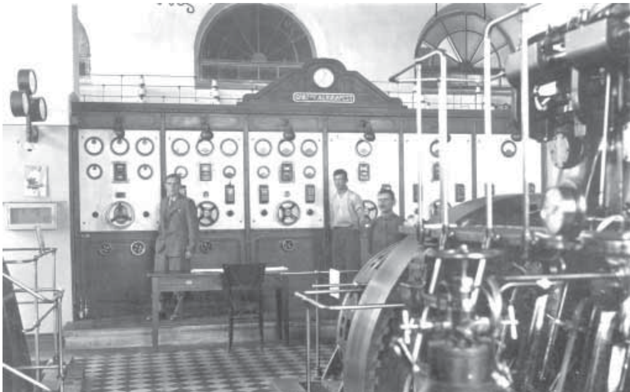
Шчытавая гарадской электрастанцыі 1930 г.. Відна марка фірмы "Ganz" і слова "Budapest".
