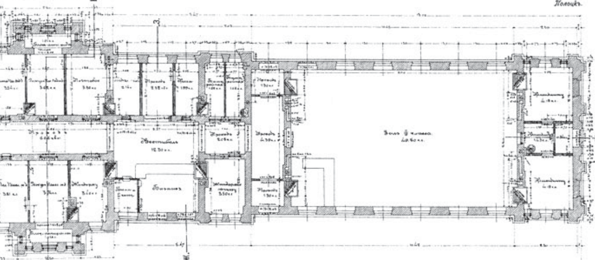
ПЛАНЪ СТѢНЪ.
