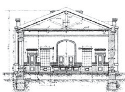
ПОПЕРЕЧНЫЙ РАЗРѢЗЪ ПО В-Г.
