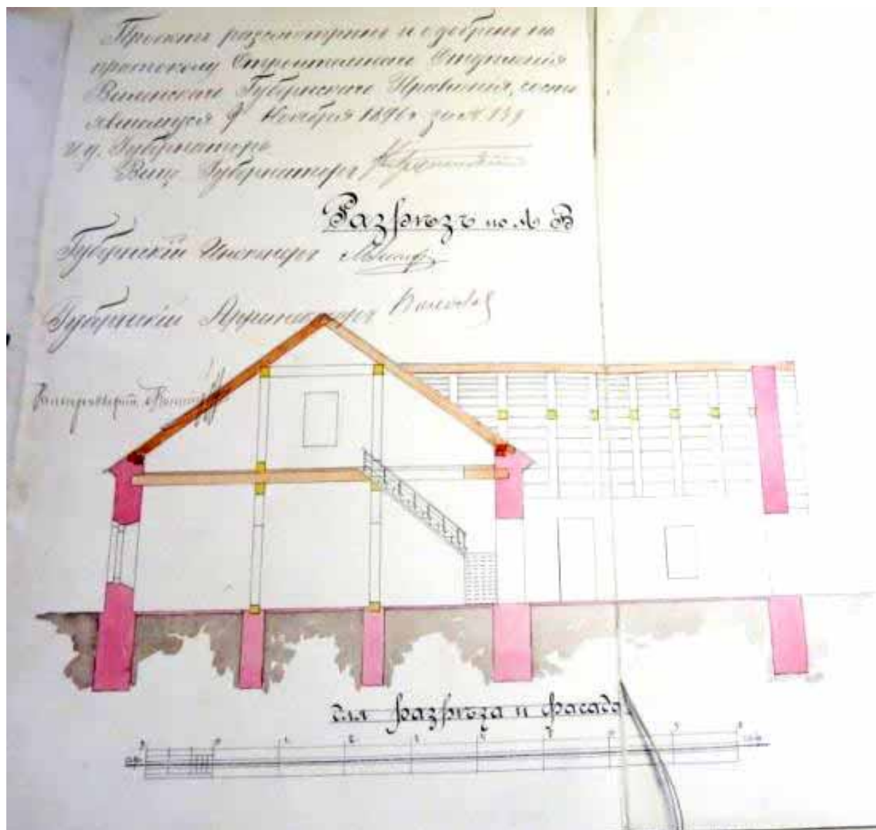
Праект крухмальнага завода ў маёнтку Дворышча. Разрѣз у вертыкальнай плоскасці (17. Л.2)
