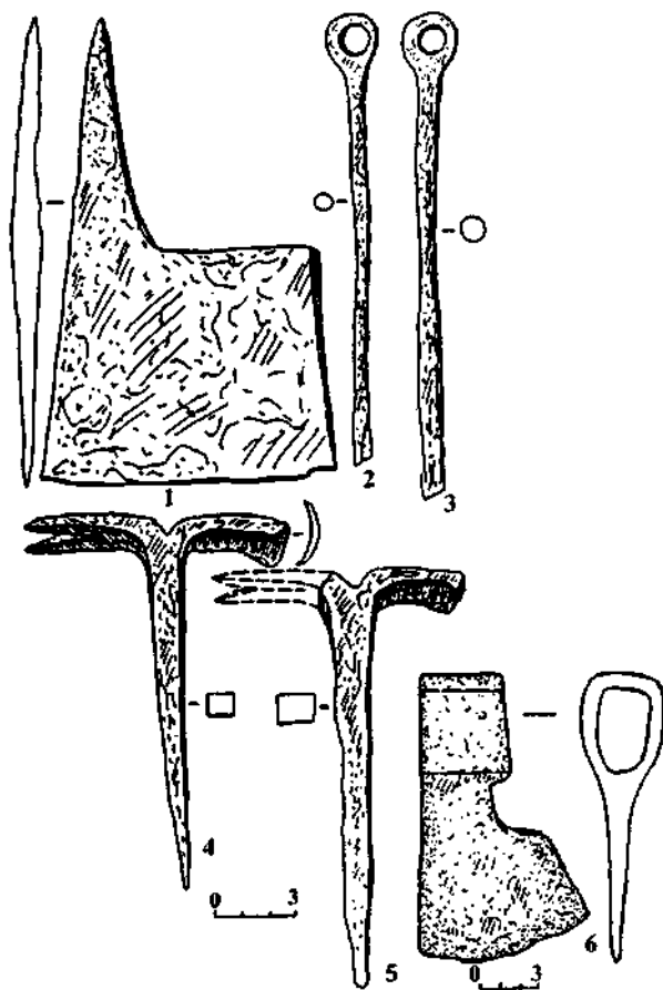
Мал. 75. Гарадзішча Замкавая гара. Дрэваапрацоўчы інструмент: 1 — фрагмент ляза сякеры; 2, 3 — свердзелы; 4, 5 — цёслы; 6 — сякера
