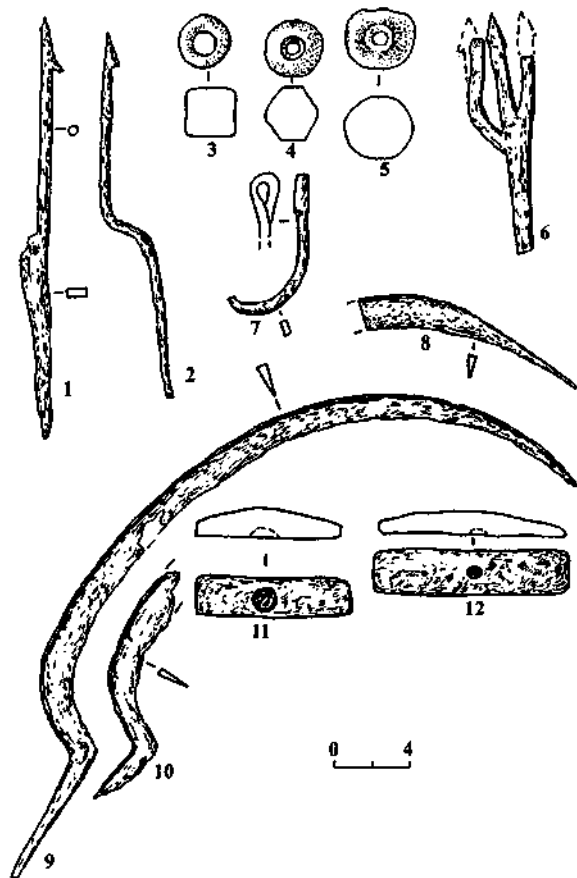
Мал. 79. Гарадзішча Замкавая гара. Сельскагаспадарчыя прылады працы і прадметы рыбалоўнага промыслу: 1, 2, 6 — восці; 3 — 5 — грузілы сетак; 7 — кручок; 8—10 — сярпы; 11, 12 — порхліцы
