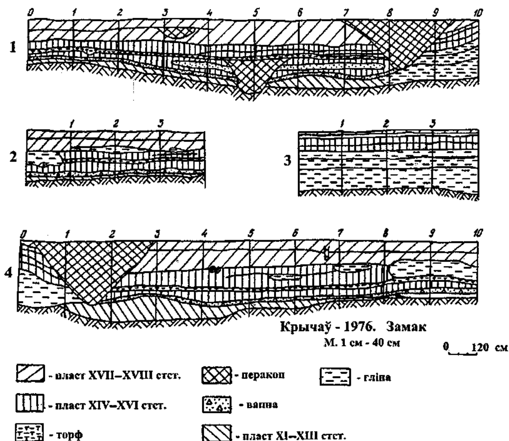
Мал. 34. Гарадзішча Замкавая гара. Профілі раскопу 1976 г. паводле М. А. Ткачова: 1 — паўночная сцяна; 2 — заходняя сцяна; 3 — усходняя сцяна; 4 — паўднёвая сцяна
