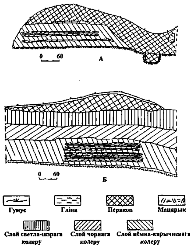
Мал. 18—19. Гарадзішча Гарадзец. Профілі раскопаў са слядамі падлог пабудовы: А — падлогі пабудовы № 1 і 2; Б — падлогі пабудовы № 6
