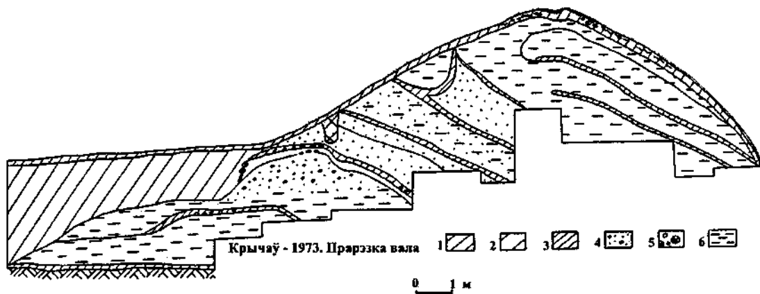
Мал. 35. Гарадзішча Замкавая тара. Прарэзка вала паводле М. А. Ткачова: 1 — дзірван; 2 — слой з матэрыяламі XII—XIII стст.; 3 — праслойкі культурнага слоя; 4 — пясок; 5 — бяровенні; 6 — гліна
