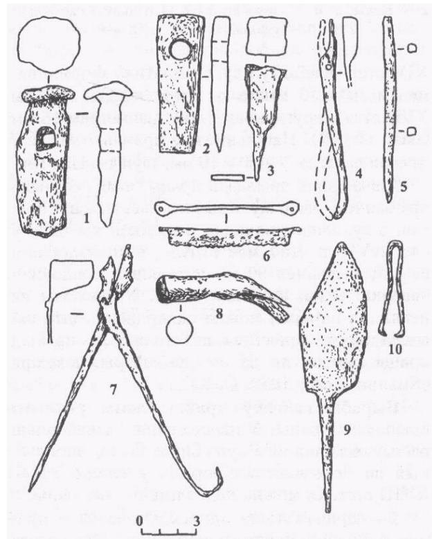
Мал. 44. Гарадзішча Замкавая гара. Інструментарый: 1 — 2 — зубіла; 3 — кавадла; 4, 7 — кузнечныя абцугі; 5 — прабойнік; 6 — пілка; 8 — малаток; 9 — нож; 10 — пінцет
